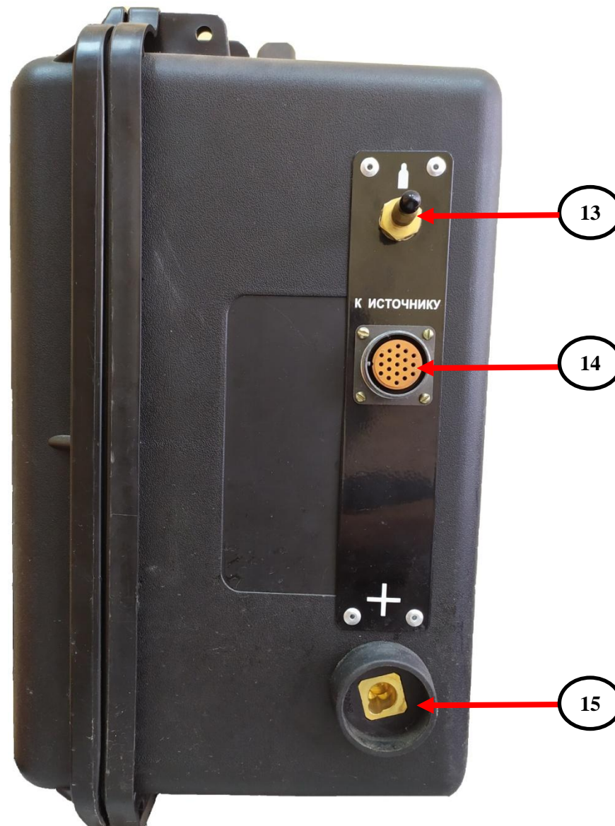
Рис.5 Задняя панель.
