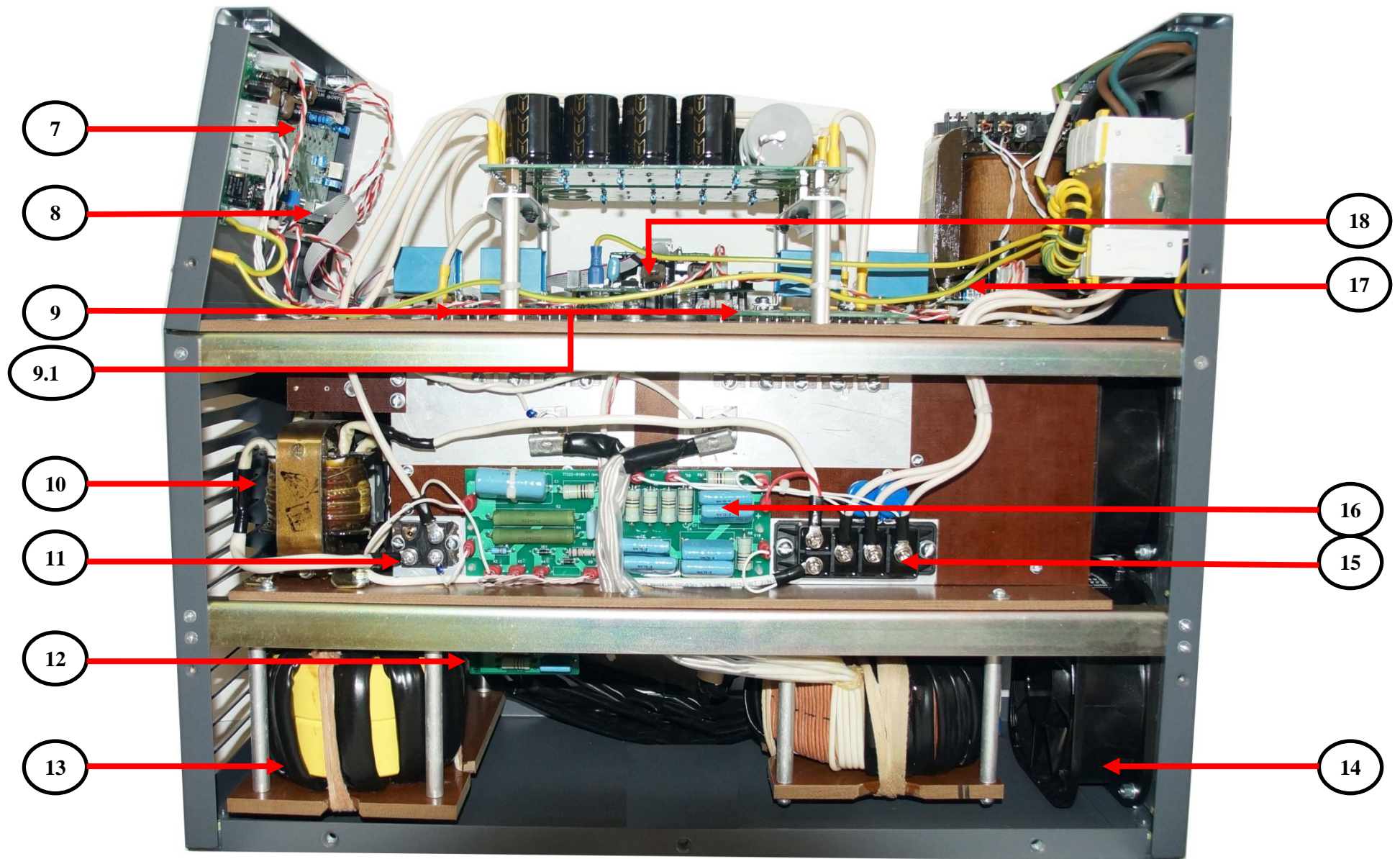
Рис.7 Вид справа.
