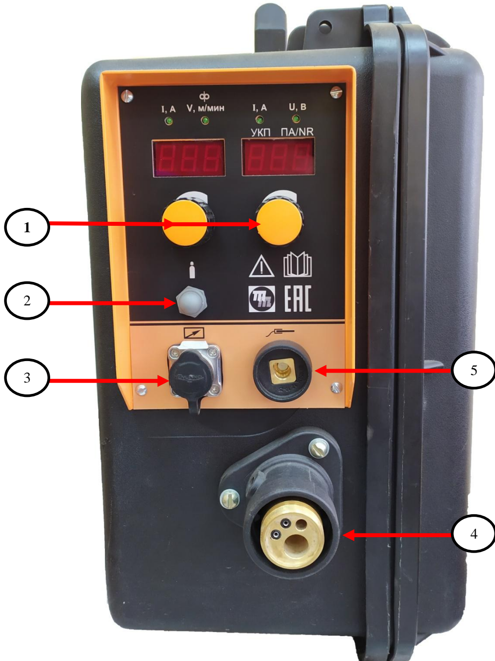
Рис.3 Передняя панель.
