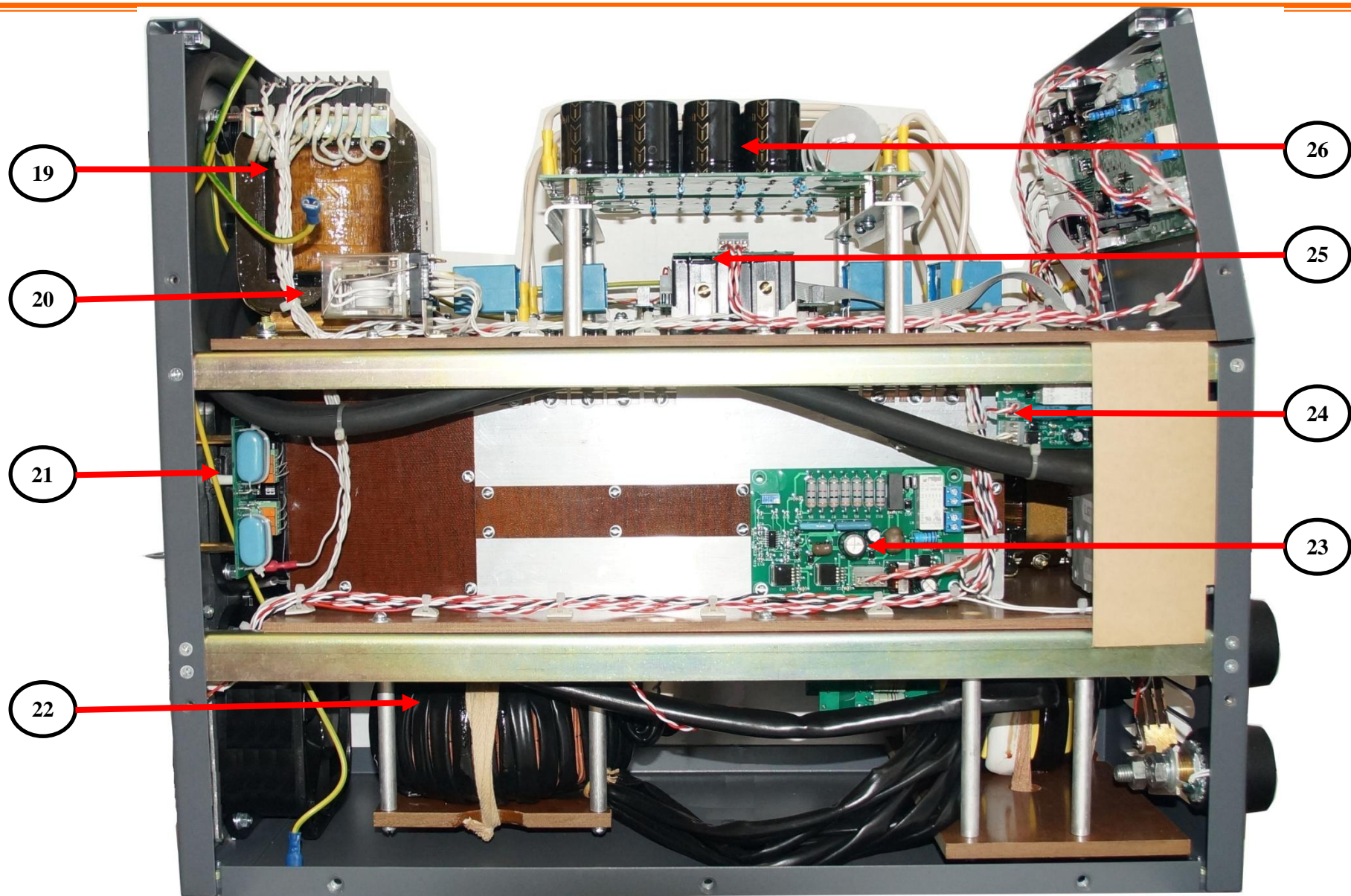
Рис.8 Вид слева.
