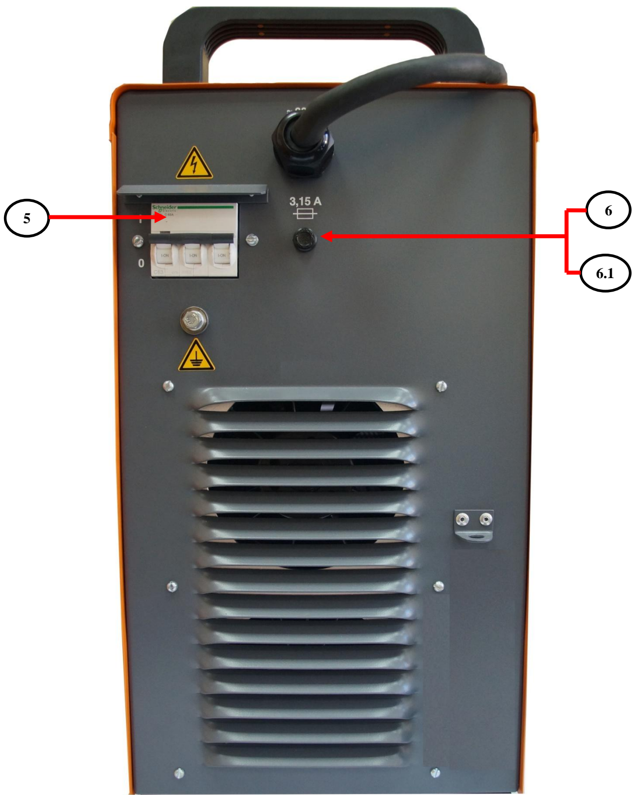
Рис.6 Задняя панель.
