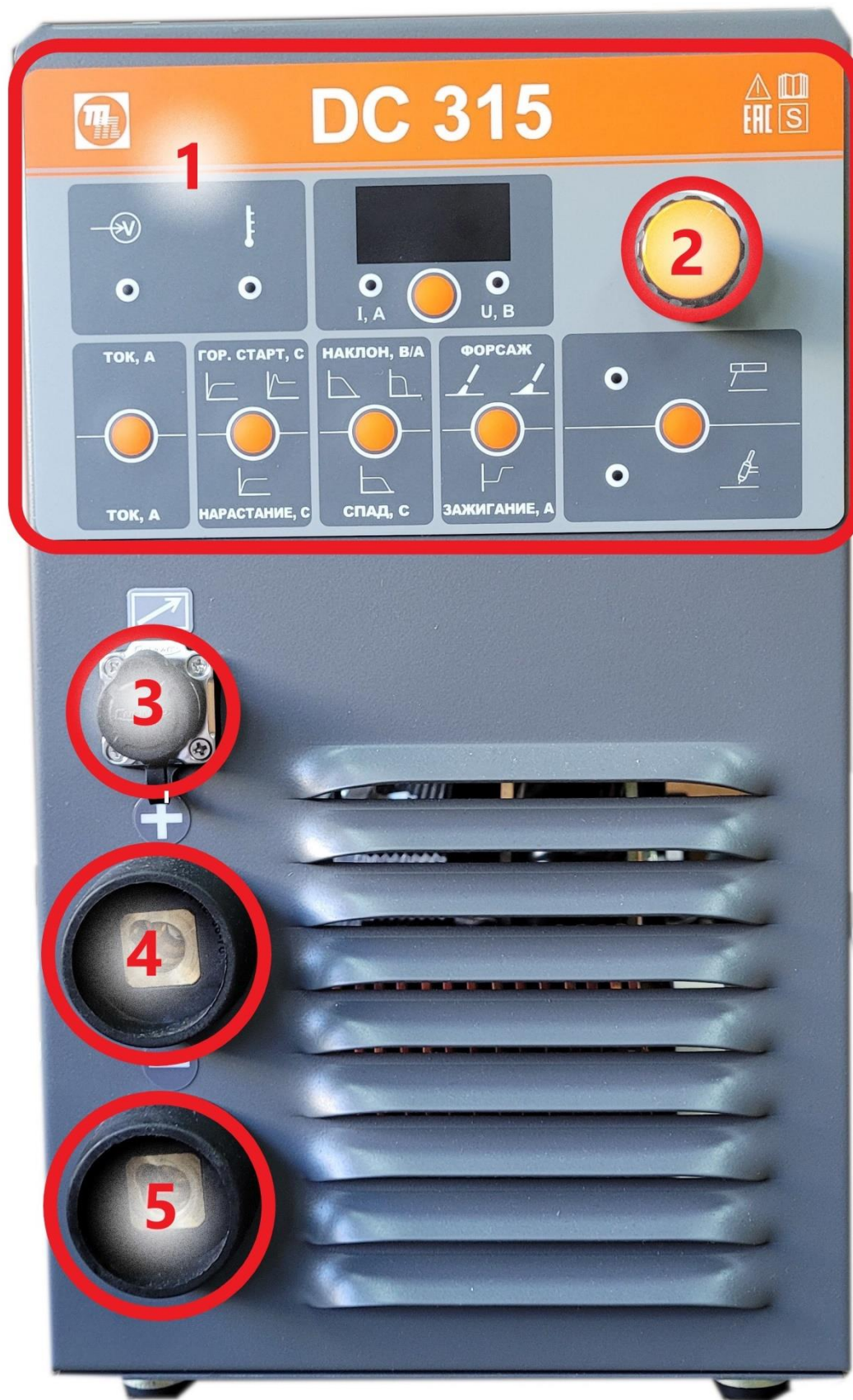
Рис.1 Передняя панель.
